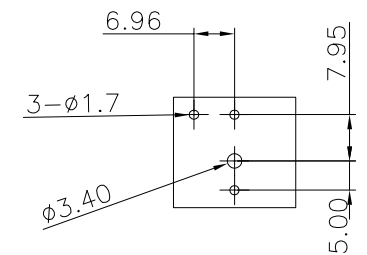
P.C.B Layout ( 1 : 1 )
