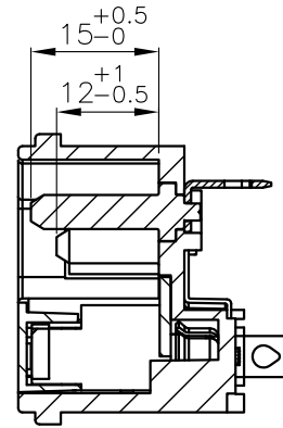
剖面圖 A-A
